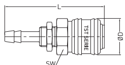
Panel Mount Standard Hose Coupling Kupplung mit Schottverschraubung Schlauchanschluss
