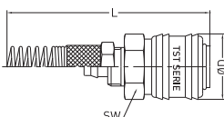
Plastic Hose Coupling With Spring Kupplungen für Kunststoffschlauch mit Knickschutzfeder
